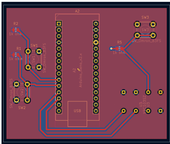
( F.Cu & B.Cu ) Panel
