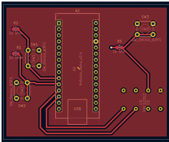
Front face (F.Cu) - VDD
