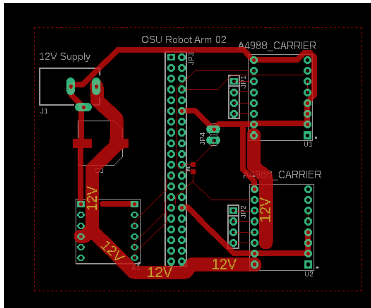
Figure 4: Top layer and silkscreen, no copper pour
