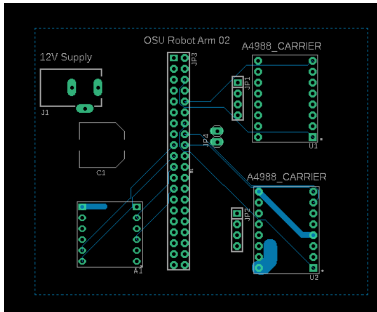
Figure 6: Bottom layer and silkscreen, no copper pour
