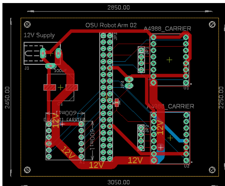
Figure 2: All layers, no copper pour
